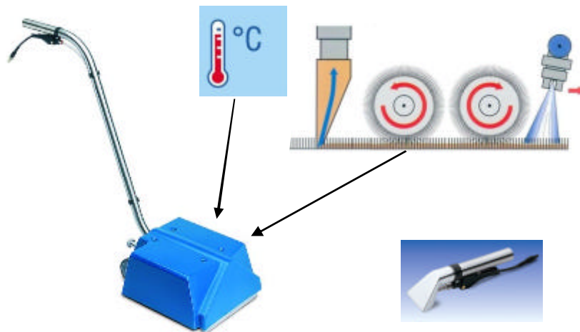
Accessoire chauffant avec brosse NS400BR-HT avec réchauffeur instantané de l'eau situé à l'intérieur
